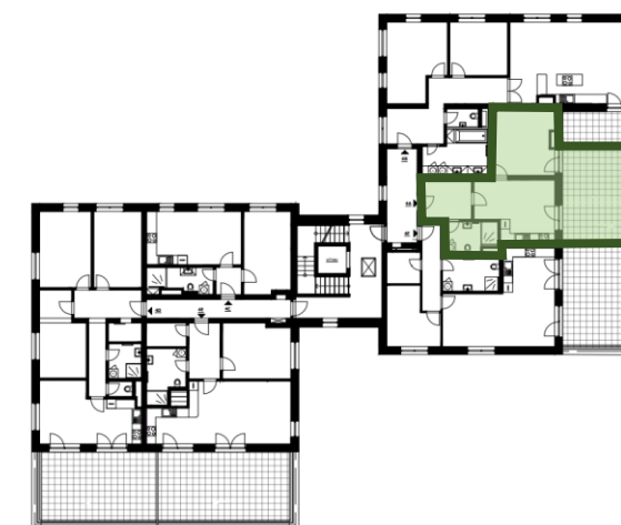
PŮDORYS PODLAŽÍ
