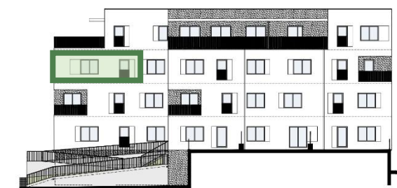
POHLED JIHOZÁPADNÍ
