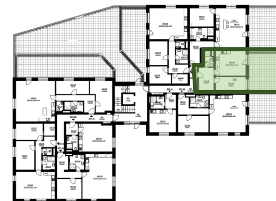
PŮDORYS PODLAŽÍ
