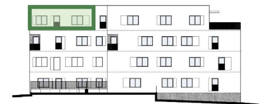
POHLED SEVEROVÝCHODNÍ
