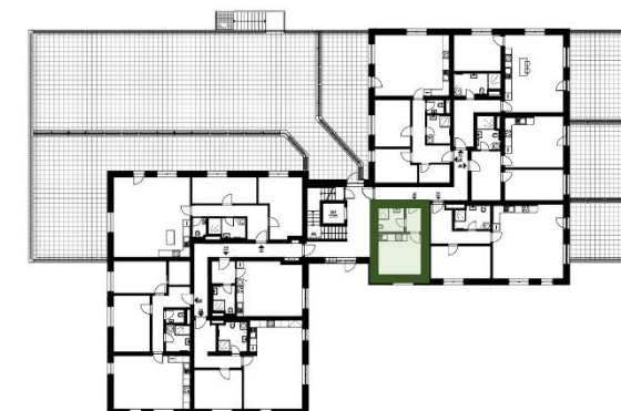
PŮDORYS PODLAŽÍ
