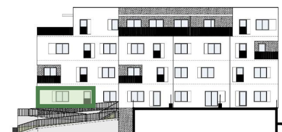
POHLED JIHOZÁPADNÍ
