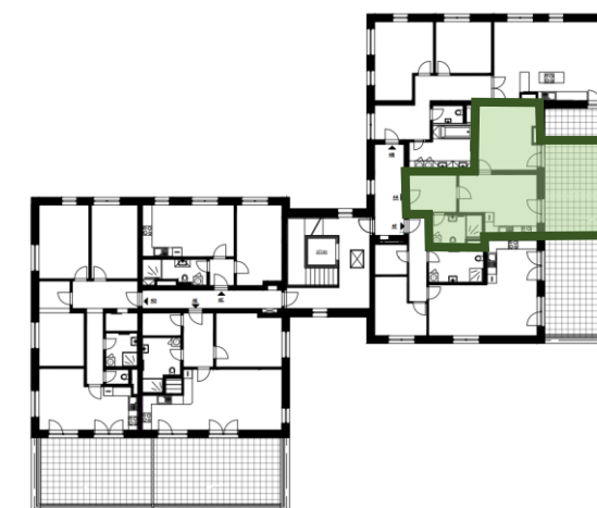
PŮDORYS PODLAŽÍ
