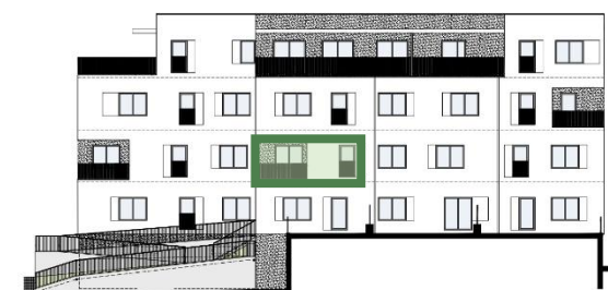
POHLED JIHOZÁPADNÍ
