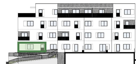
POHLED JIHOZÁPADNÍ
